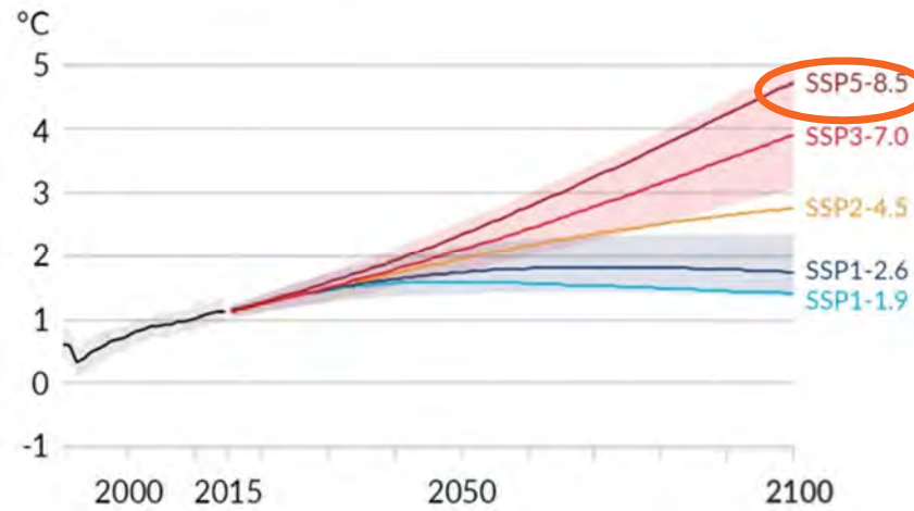
世界平均気温の変化
